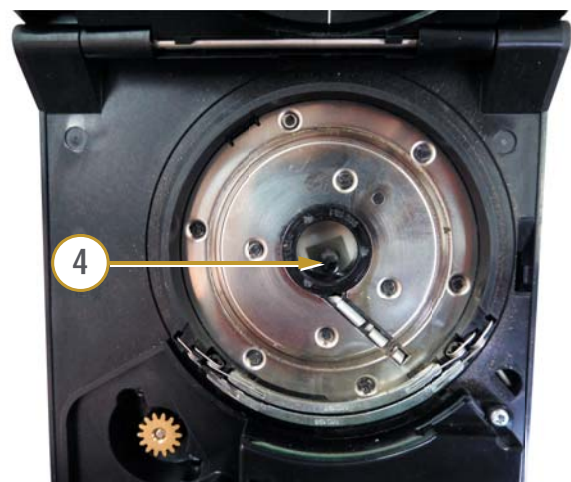
Figura 4.2.k Desmontaje Disco 4
