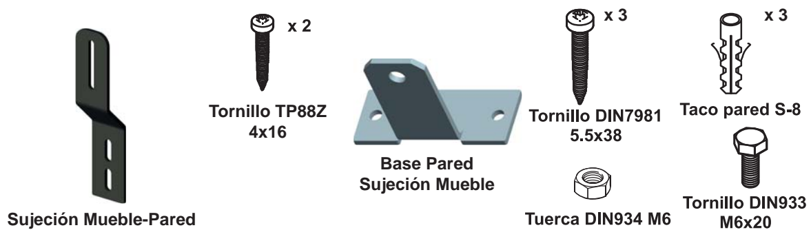
Figura 1.6.a Material Fijación
