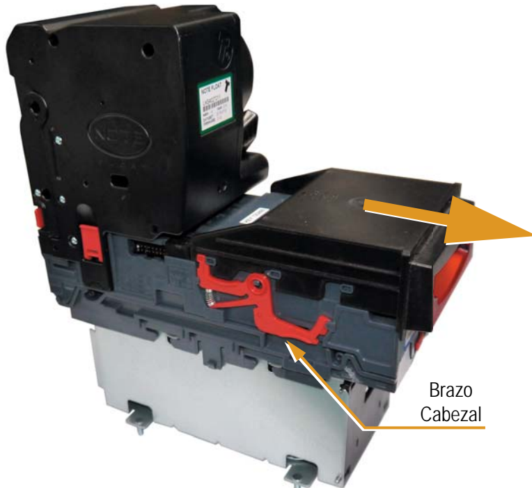
Figura 4.1.h Extracción cabezal
