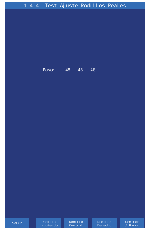
Figura 6.1.4.4. Test Ajuste Rodillos Reales
