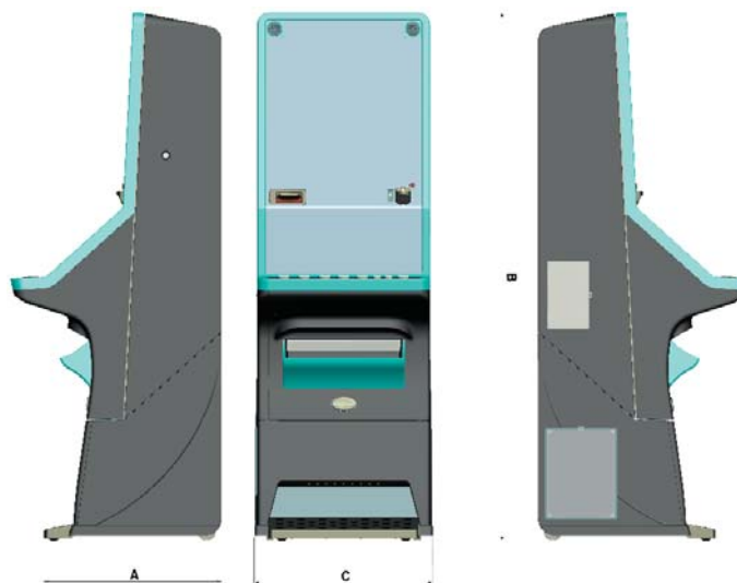
Figura 3.1.1 Dimensiones
