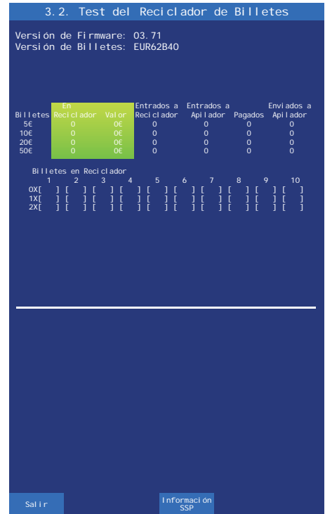
Figura 6.3.2a Test del Reciclador de Billetes
